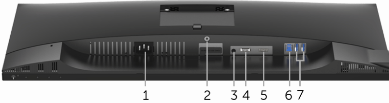
Ansicht von unten ohne Monitor-Standfuß
